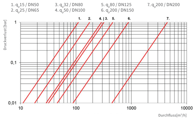
Typische Druckverlustkurve
